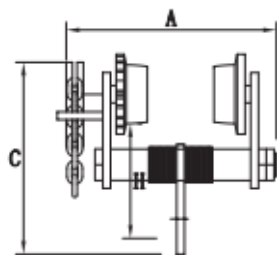
1/2-20т приводная тележка
