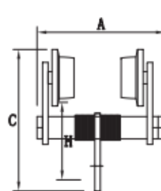
1/2-10т холостая тележка
