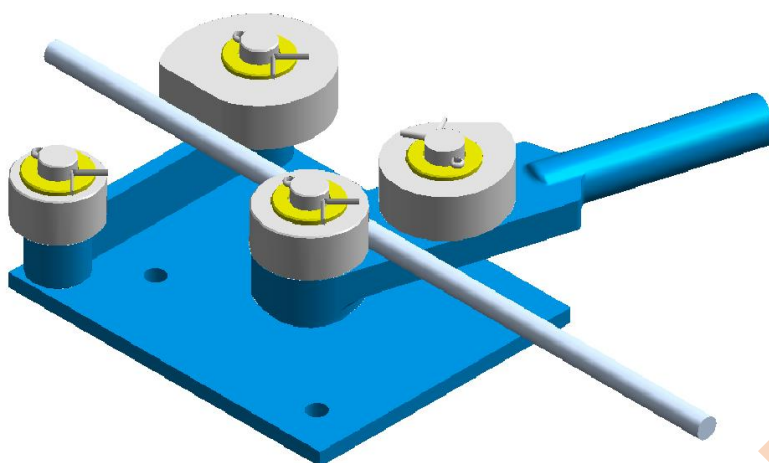
Расположение прута в гибочных машинах DR-25
